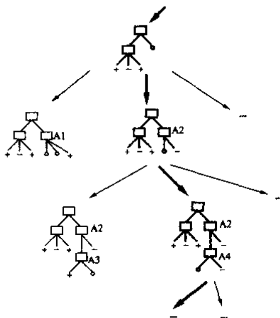
ID3 遍历可能决策树的空间,从最简单的树到逐渐复杂的树,其搜索由信息增益启发式规则引导
