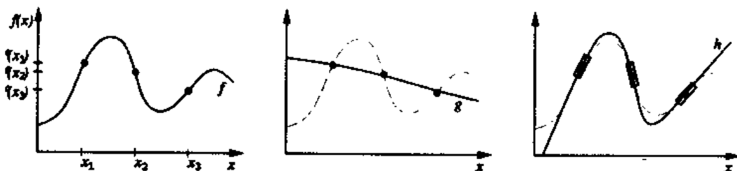
图 12-5 用 TANGENTPROP 拟合值和导数
